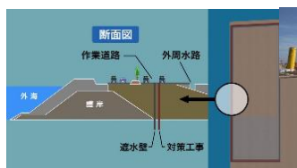
既存の遮水壁補強工事
